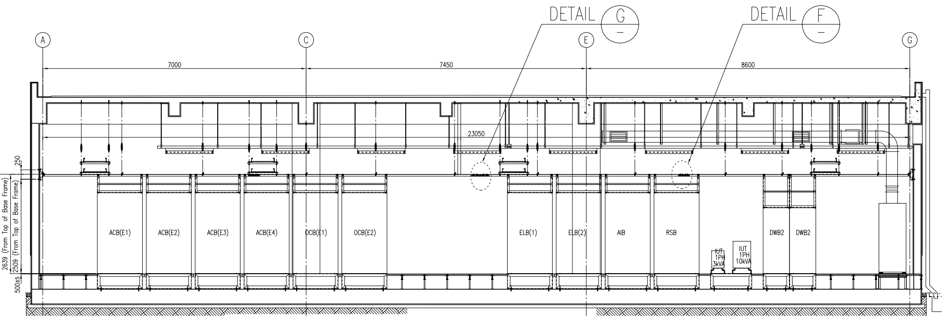
SECTION D S=1:50 0528
