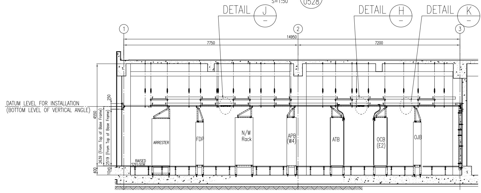
SECTION E S=1:50 0528
