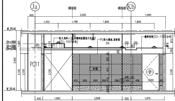
G向立面詳細圖
