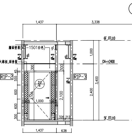
J向立面詳細圖
