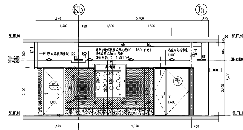
D向立面詳細圖
