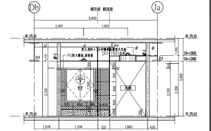
F向立面詳細圖
