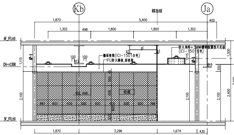
H向立面詳細圖
