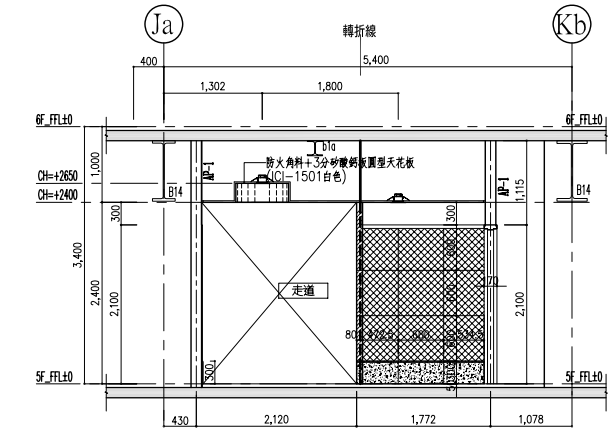
E向立面詳細圖
