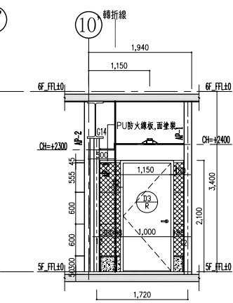
K向立面詳細圖
