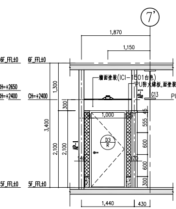
I向立面詳細圖
