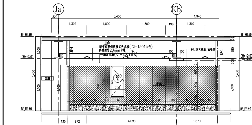
C向立面詳細圖
