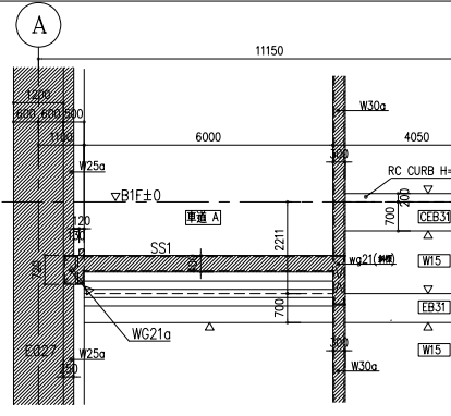
D-1 AIR SHAFT 剖面詳圖 S=1/100
