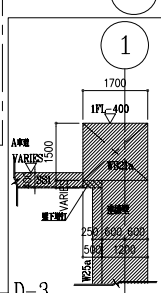
D-3 X-1 Y-A~B 剖面詳圖
