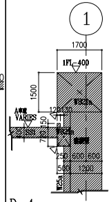
D-4 X-1 Y-B~C 剖面詳圖
