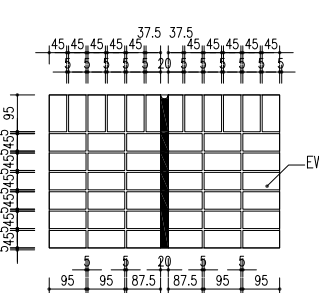
DETAIL H 詳圖 H 1:10
