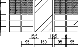
DETAIL C 詳圖 C 1:10
