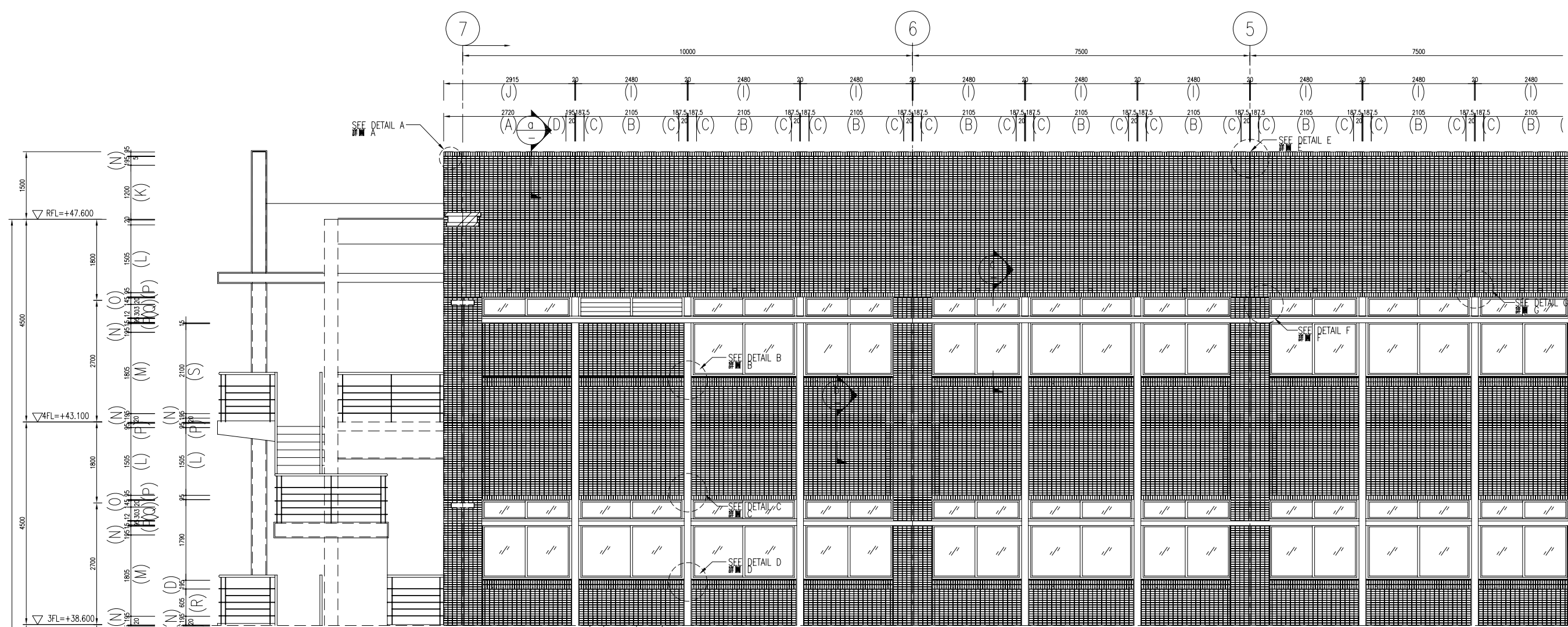
SECTION a 剖面 a 1:10
