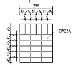
DETAIL A 詳圖 A 1:10
