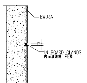
SECTION b 剖面 b 1:10
