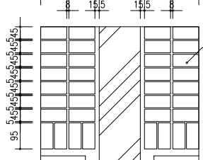
DETAIL E 詳圖 E 1:10
