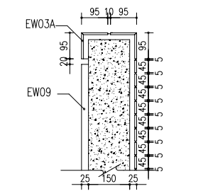
SECTION a 剖面 a 1:10
