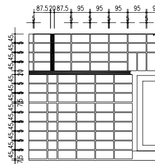
DETAIL I 詳圖 I 1:10
