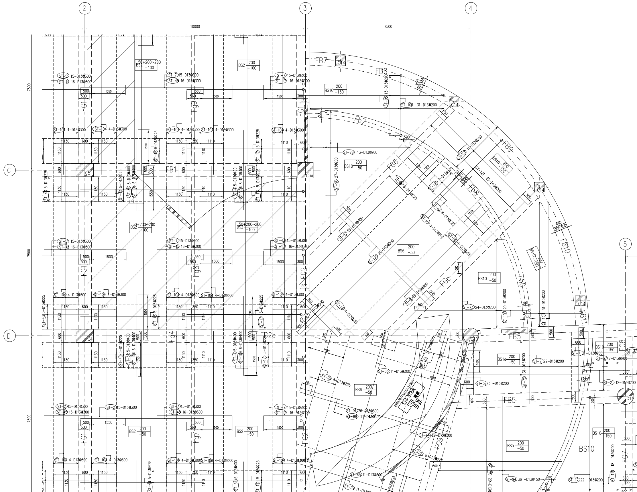
配筋平面圖 S=1/50
